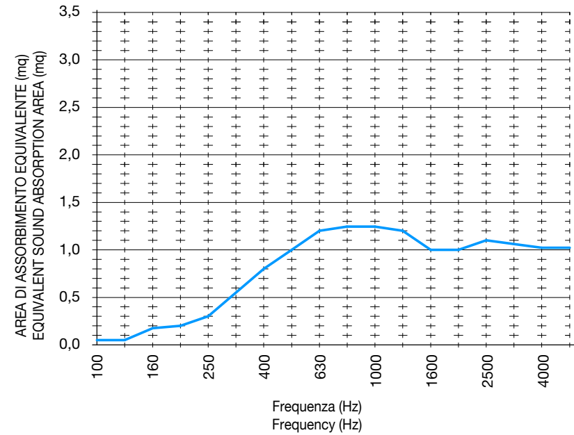
ANDAMENTO DELL'AREA DI ASSORBIMENTO ACUSTICO EQUIVALENTE Aobj PER TERZI D'OTTAVA ONE-THIRD-OCTAVE EQUIVALENT SOUND ABSORPTION AREA Aobj CURVE
