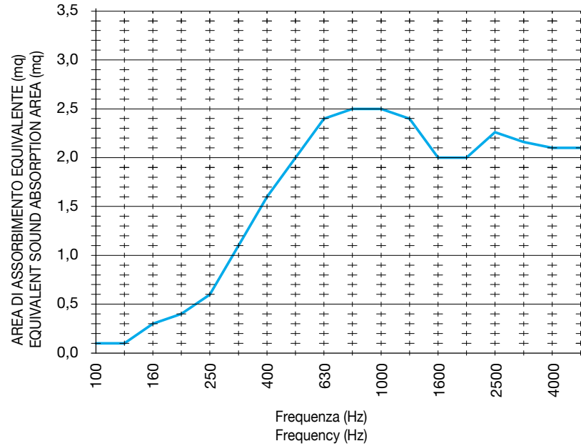
ANDAMENTO DELL'AREA DI ASSORBIMENTO ACUSTICO EQUIVALENTE Aobj PER TERZI D'OTTAVA ONE-THIRD-OCTAVE EQUIVALENT SOUND ABSORPTION AREA Aobj CURVE
